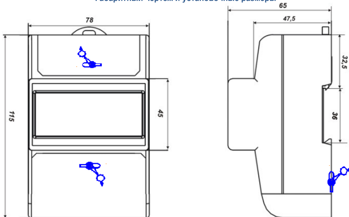
Габаритный чертеж и установочные размеры
